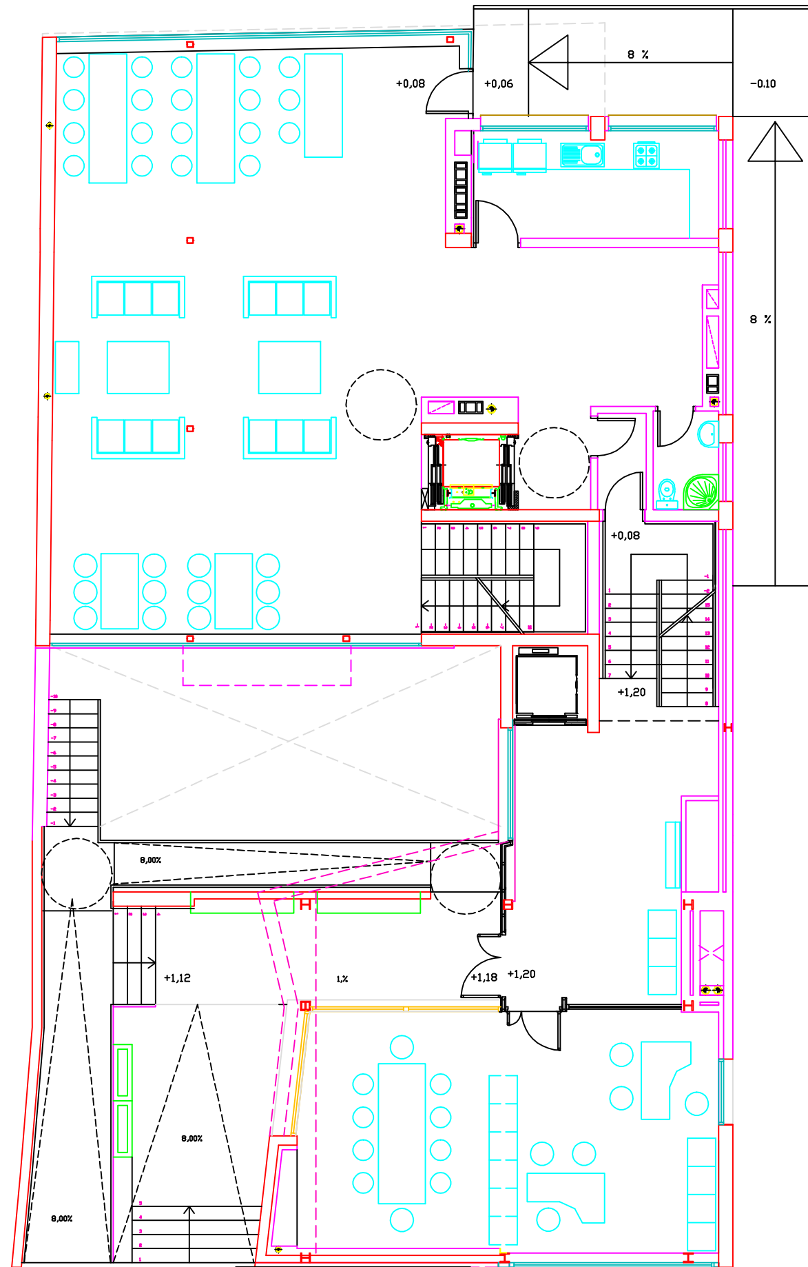
Planta Baja
